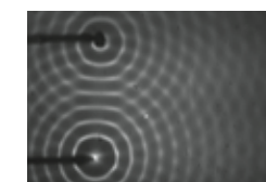
81 Zwei Erreger erzeugen Kreiswellen, die miteinander interferieren. Ein typisches Muster mit Knotenlinien entsteht.
