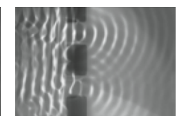
82 Eine Welle läuft vom Erreger auf einen Doppelspalt zu. Von den beiden Spaltöffnungen gehen Kreiswellen aus.
