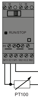
3Leitertechnik
