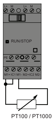
2Leitertechnik
