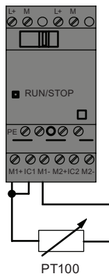
2Leitertechnik
