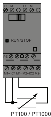
3Leitertechnik
