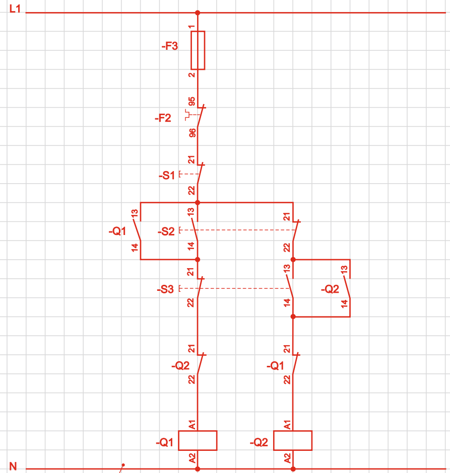
Wendeschützschtaltung mit direkter Umschaltung
