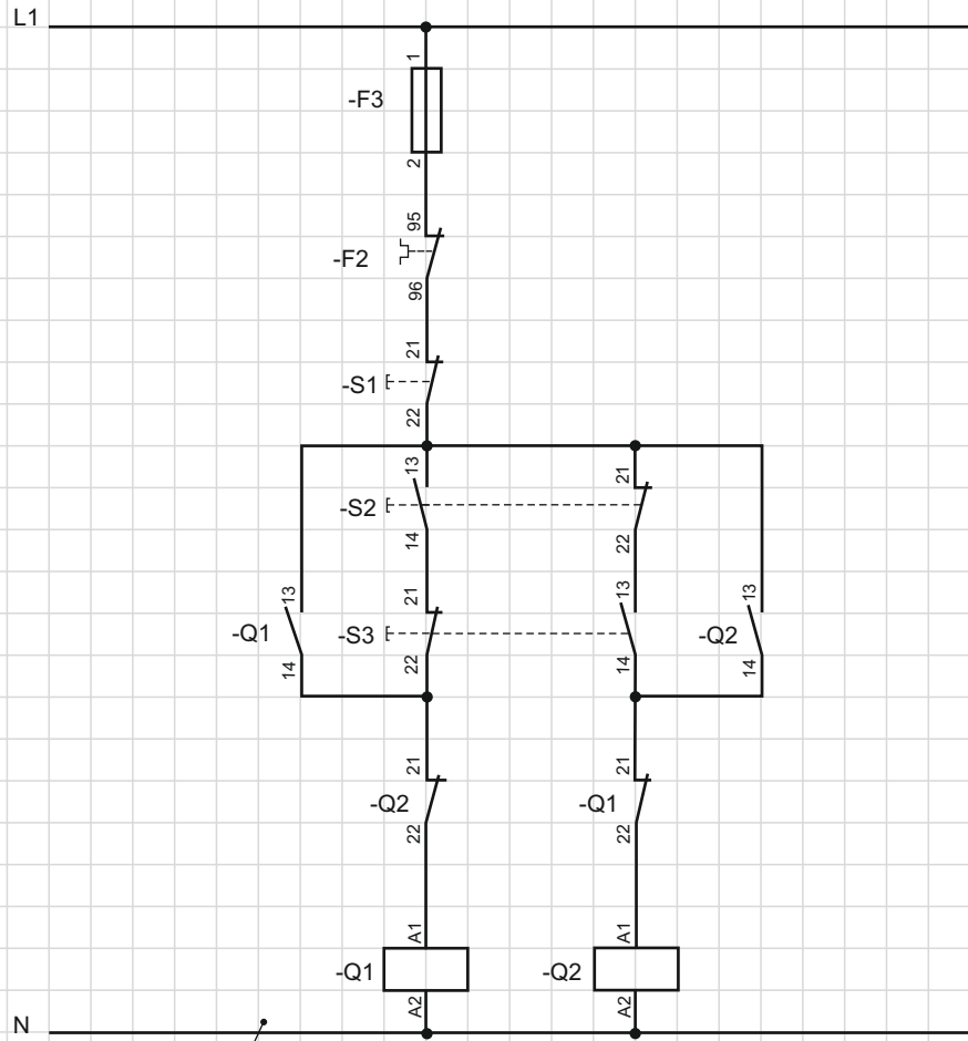
Wendeschützschtaltung mit indirekter Umschaltung
